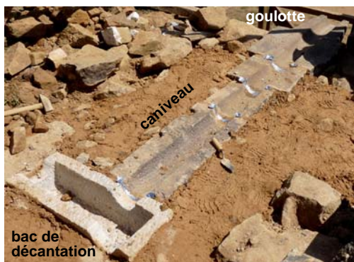
Système d'écoulement des eaux de pluie
